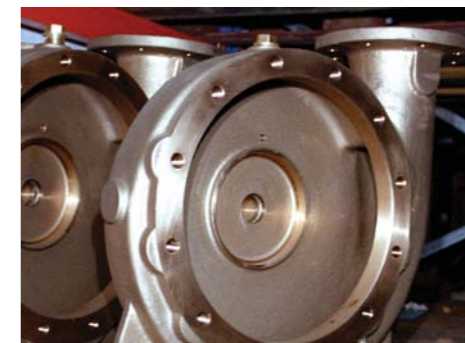
Gehäuse einer seewasserbeständigen Bronzepumpe
